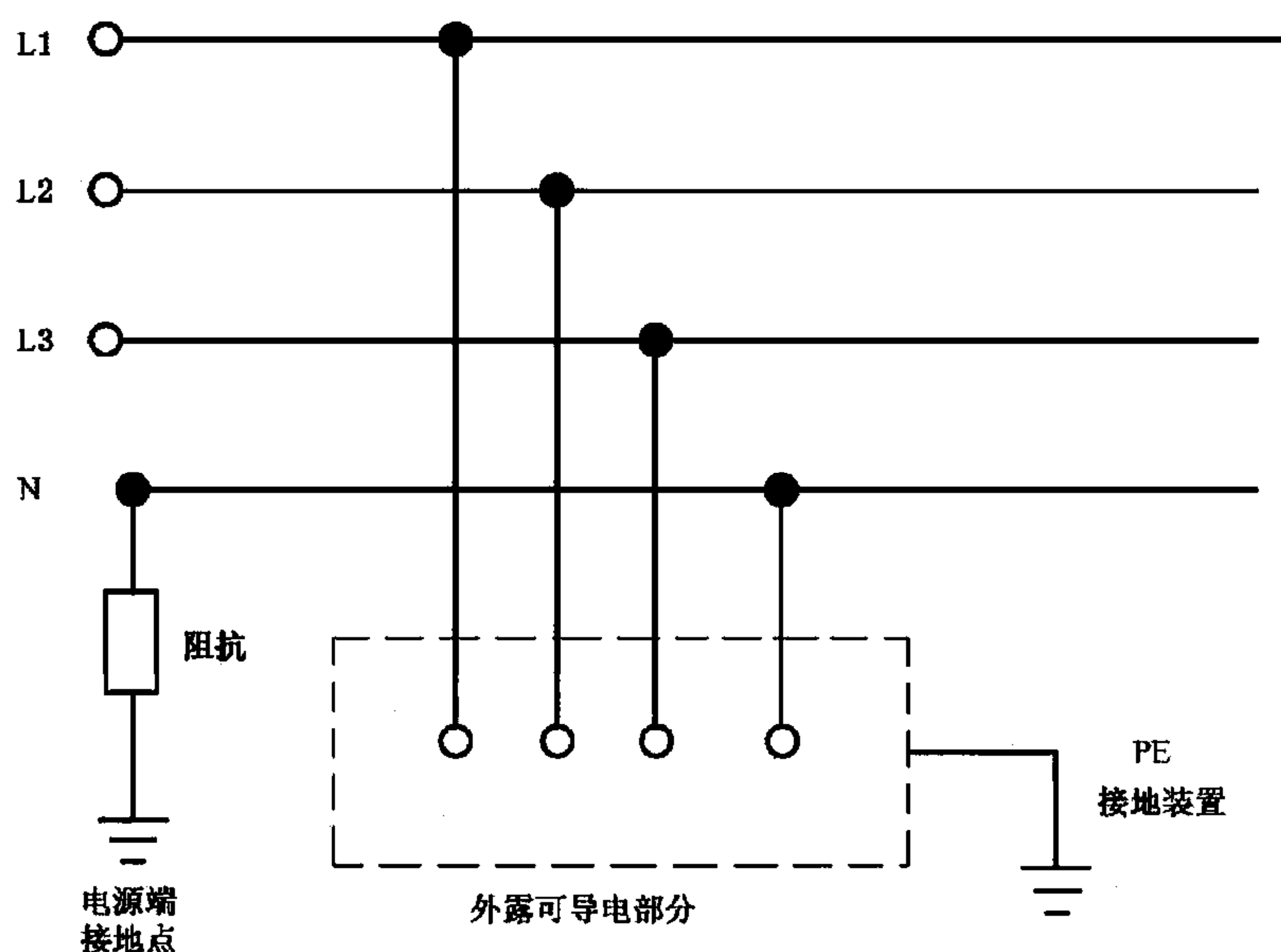
图 5 IT 系统
